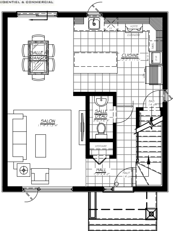
Rez-de-Chaussée
