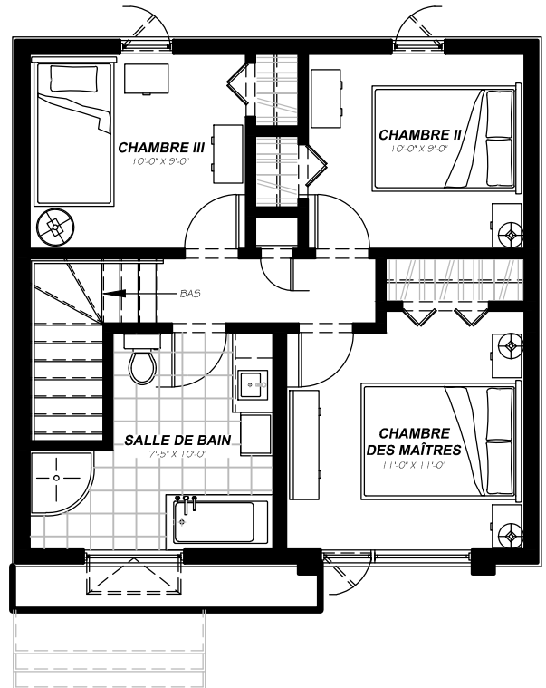
Étage
