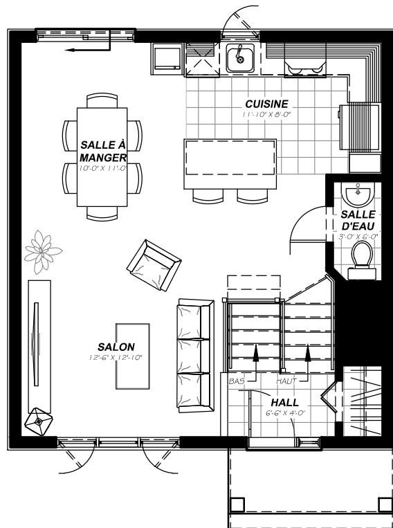
Rez-de-Chaussée
