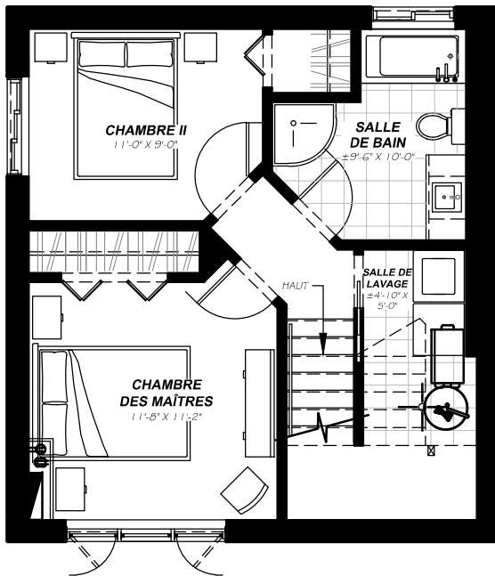
Sous-Sol
