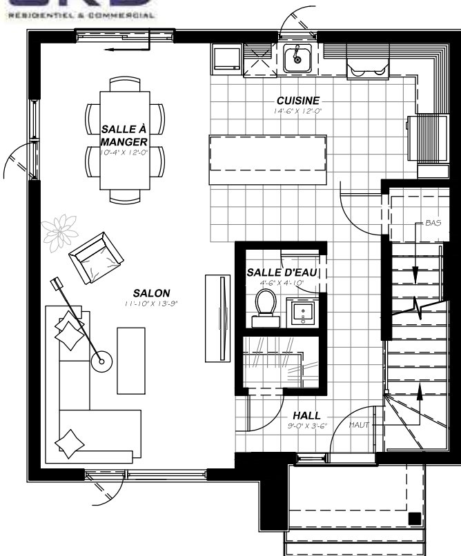
Rez-de-Chaussée
