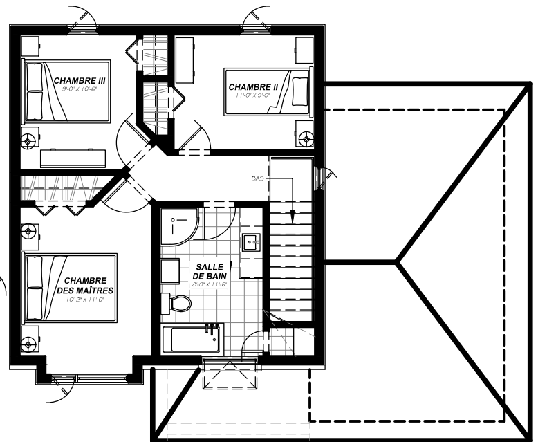
Étage
