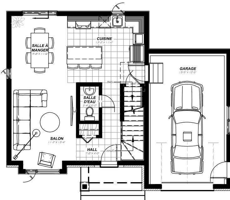
Rez-de-Chaussée
