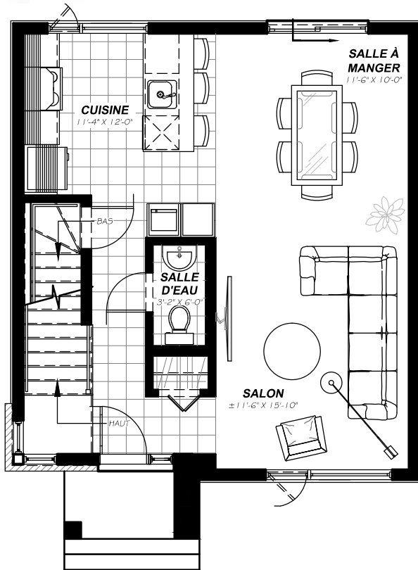
Rez-de-Chaussée
