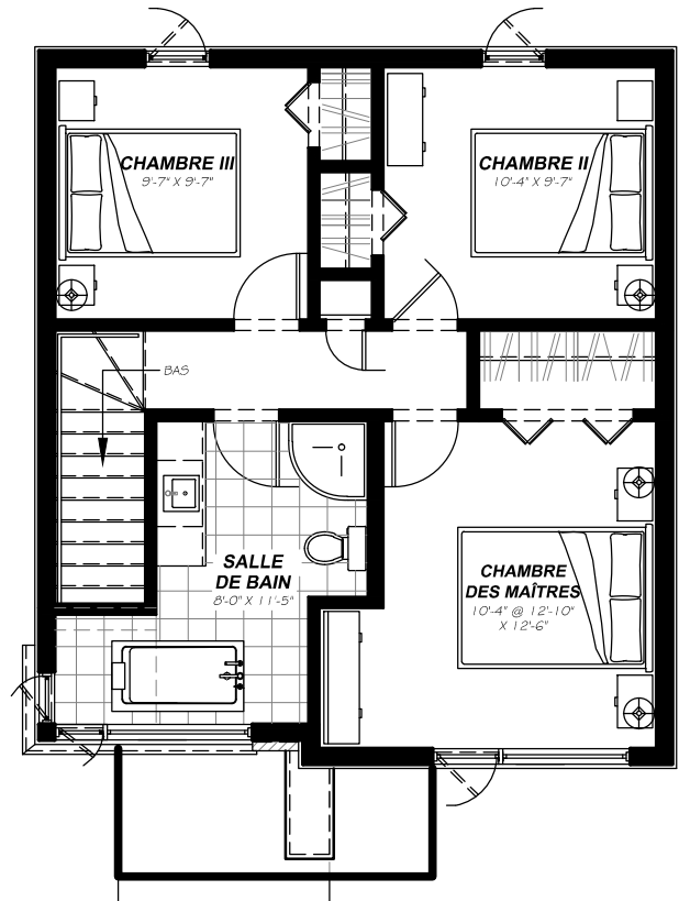
Étage
