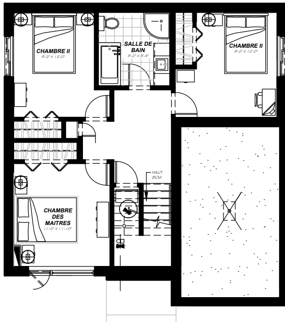
Sous-Sol
