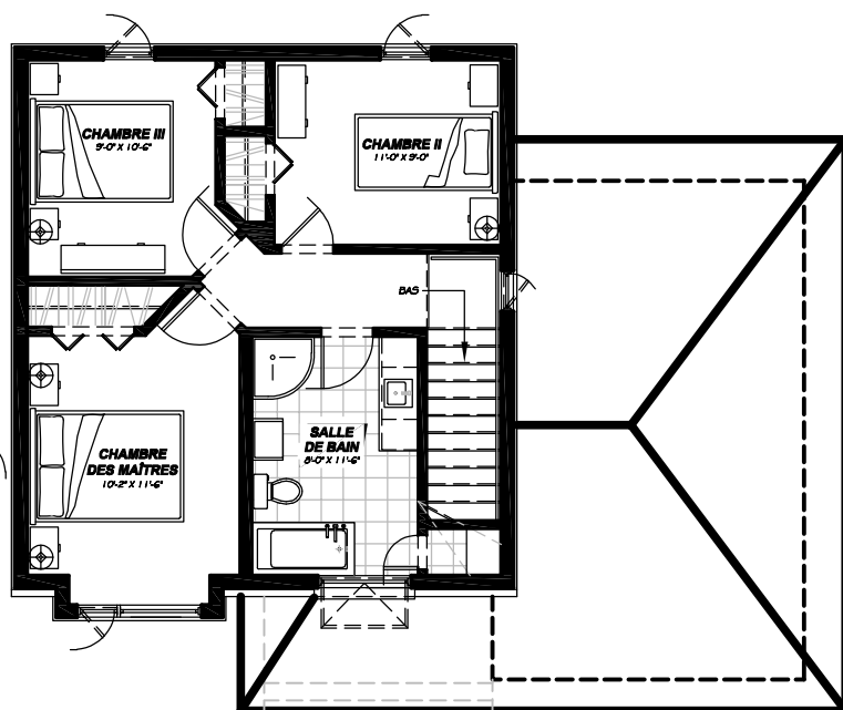
Étage
