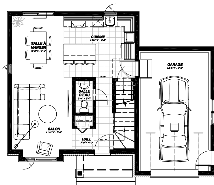
Rez-de-Chaussée
