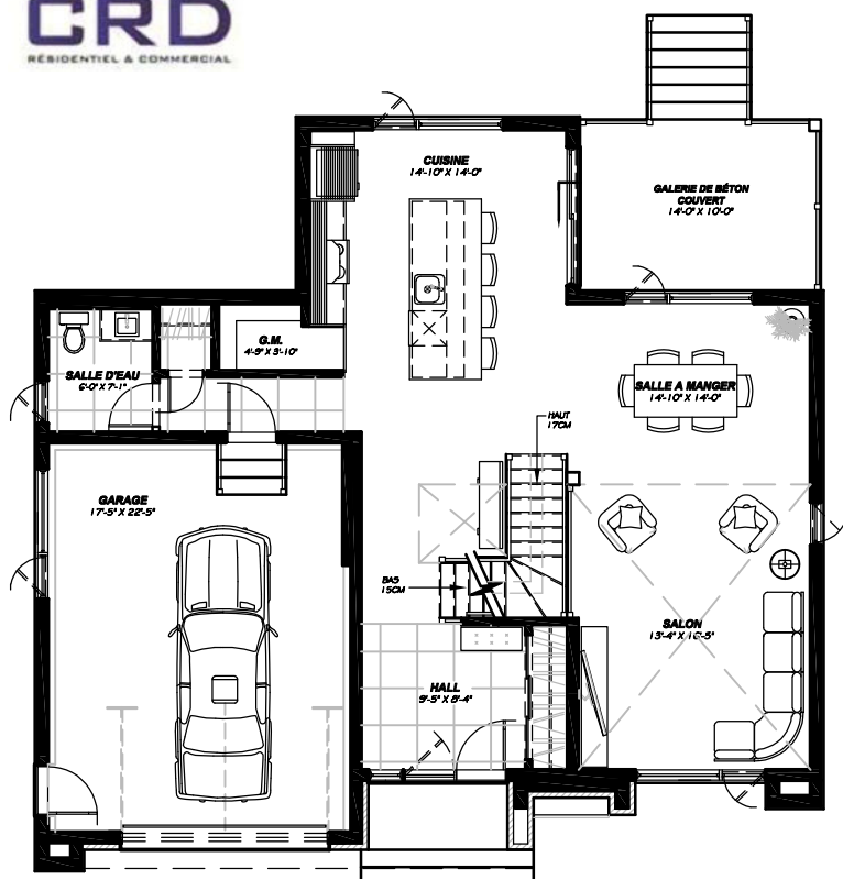
Rez-de-chaussée
